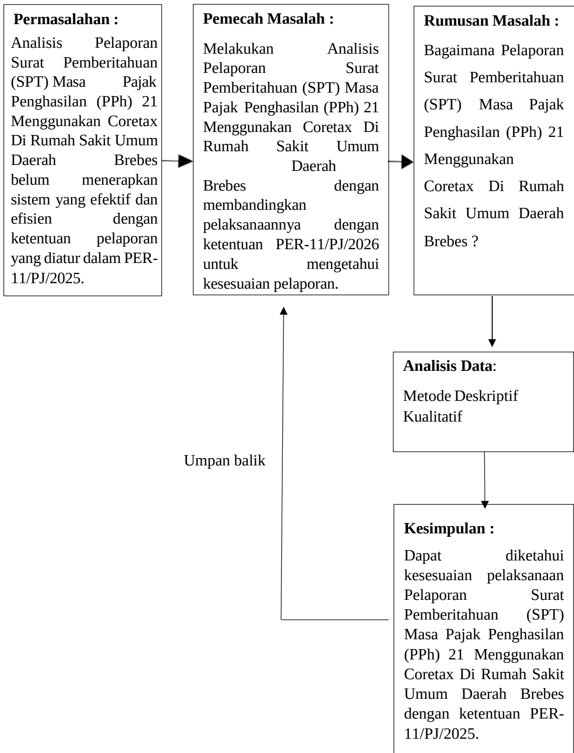
Gambar 1 Kerangka Berpikir
